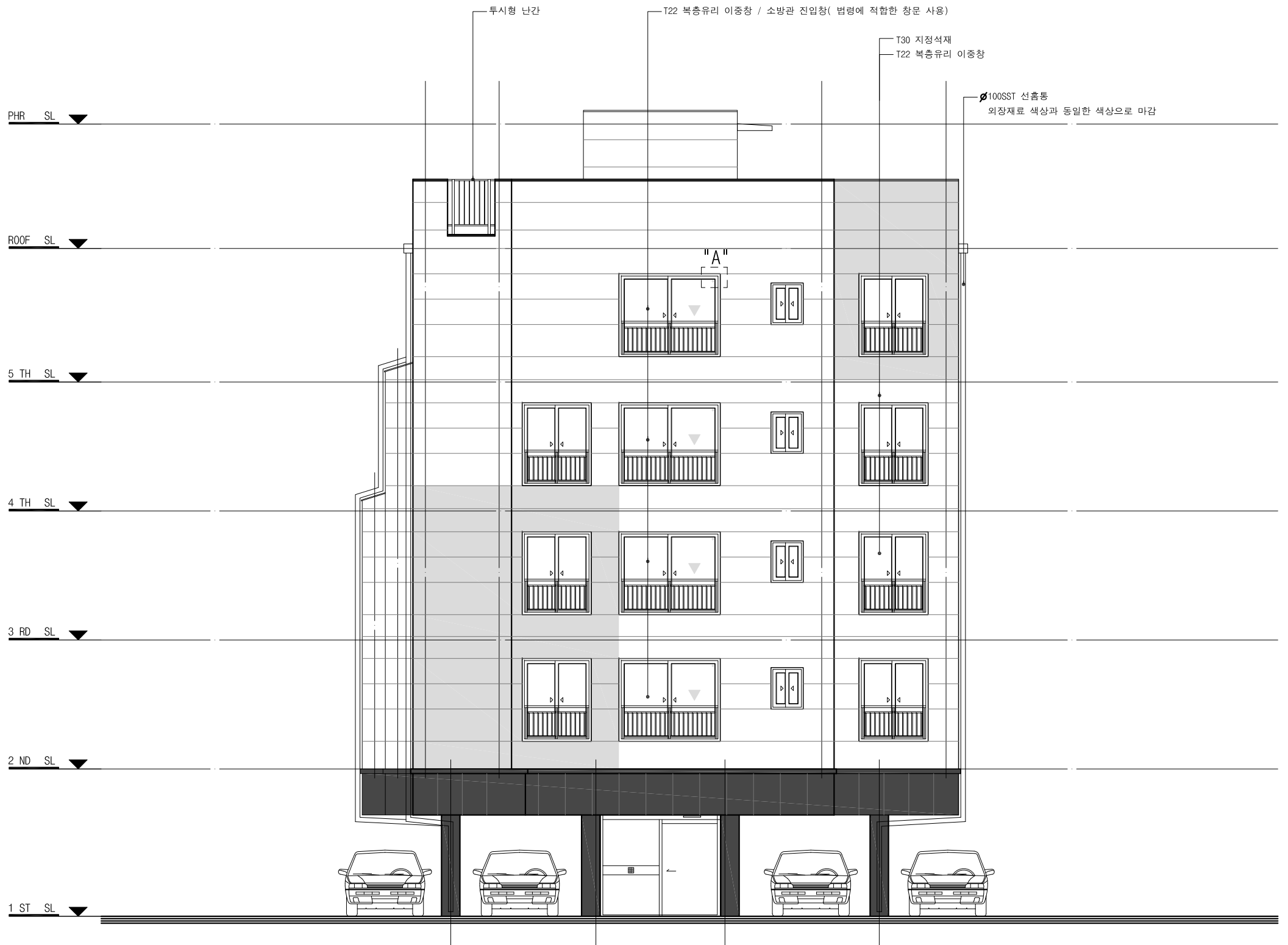
정 면 도 SCALE: 1/100
