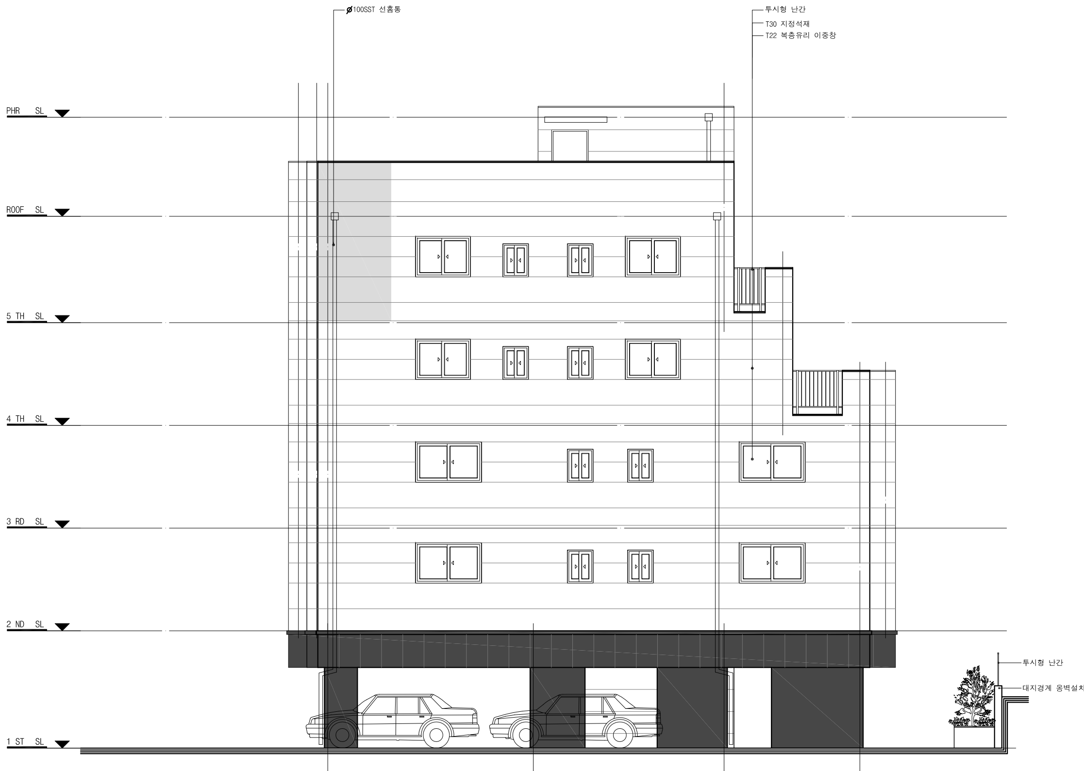
우 측 면 도 SCALE: 1/100
